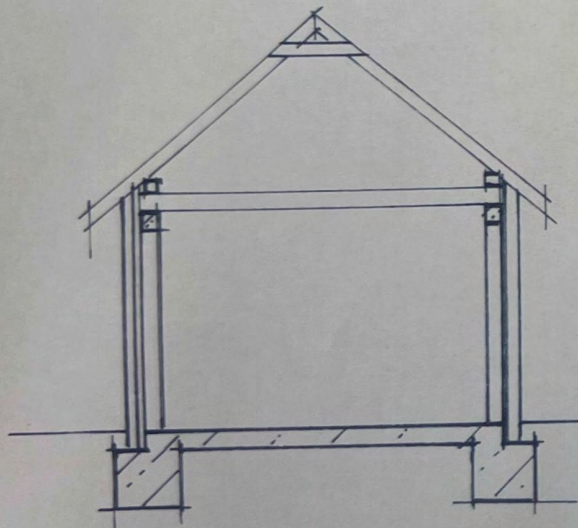
SCHNITT C-C
