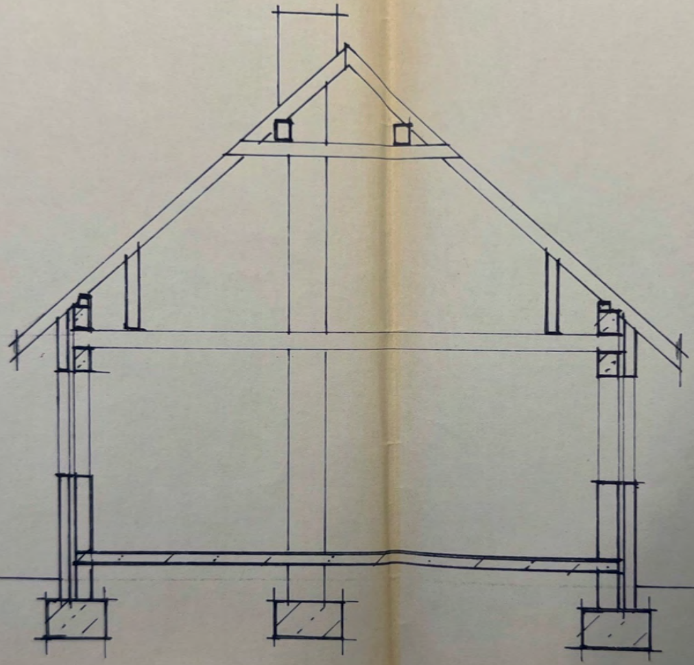
SCHNITT 3-3
